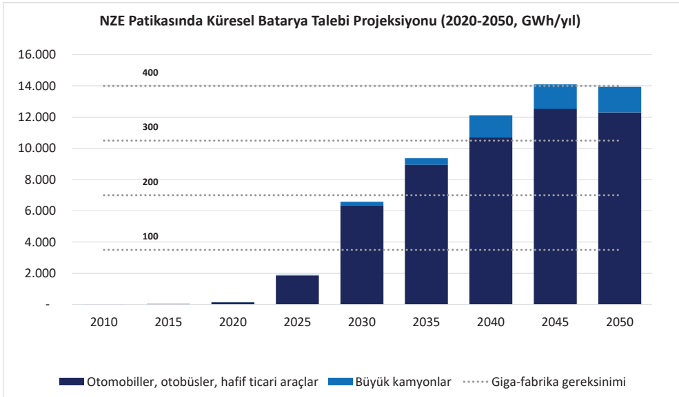
Şekil 3.32. NZE Patikasında Küresel Batarya Talebi Projeksiyonu (2020-2050, GWh/yıl)
