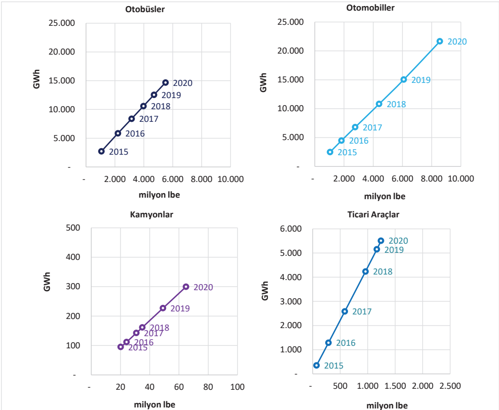
Şekil 3.24. Küresel Ölçekte EA Türleri Bazında Yıllık Petrol Tüketiminde Tasarruf ve Elektrik Talebi Gelişimi (2015-2020, mİbe ve GWh)
