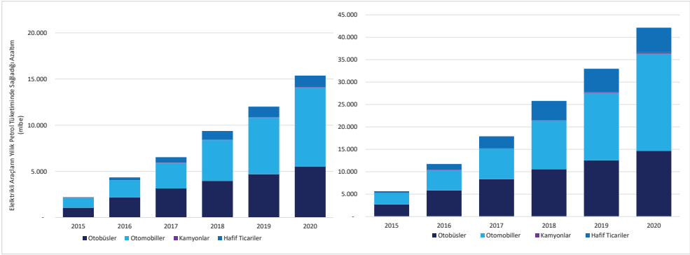
Şekil 3.23. Küresel Ölçekte EA Türleri Bazında Yıllık Petrol Tüketiminde Tasarruf ve Elektrik Talebi Gelişimi (2015-2020, mİbe ve GWh)
