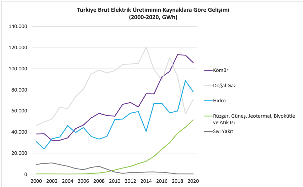
Şekil 4.24. Türkiye Brüt Elektrik Üretiminde Gelişimi ve Yenilenebilir Enerjinin Katkısı (2010-2020, GWh, %)
