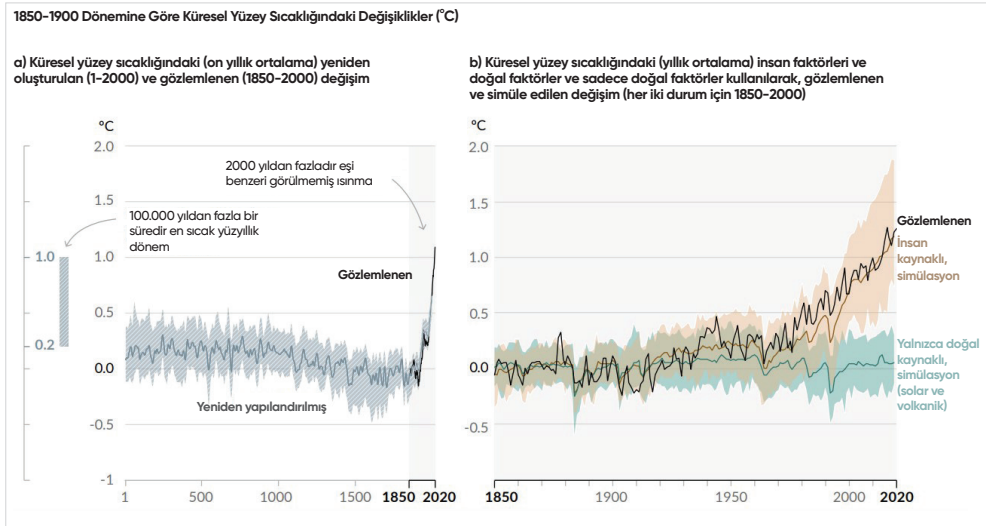
Şekil 2.2. Dönemine Göre Küresel Yüzey Sıcaklığındaki Değişiklikler (°C)
